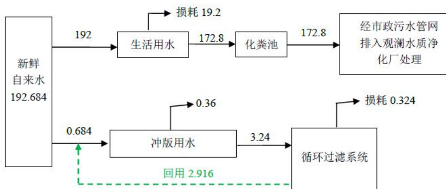
图 4-2 项目水平衡图 单位 t/a
